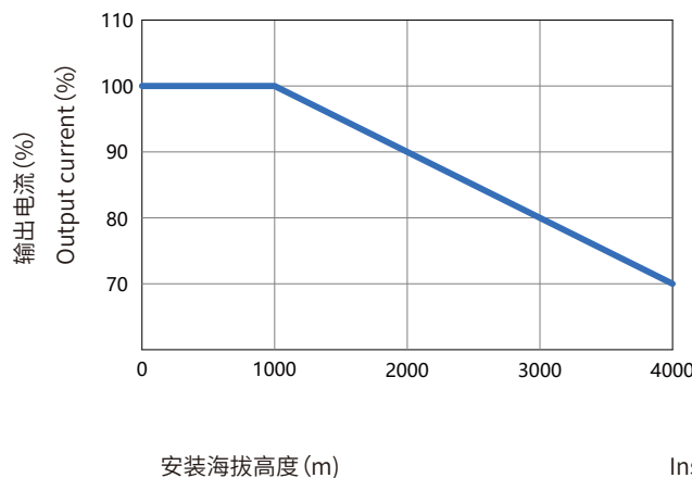
降容数据·海拔高度
